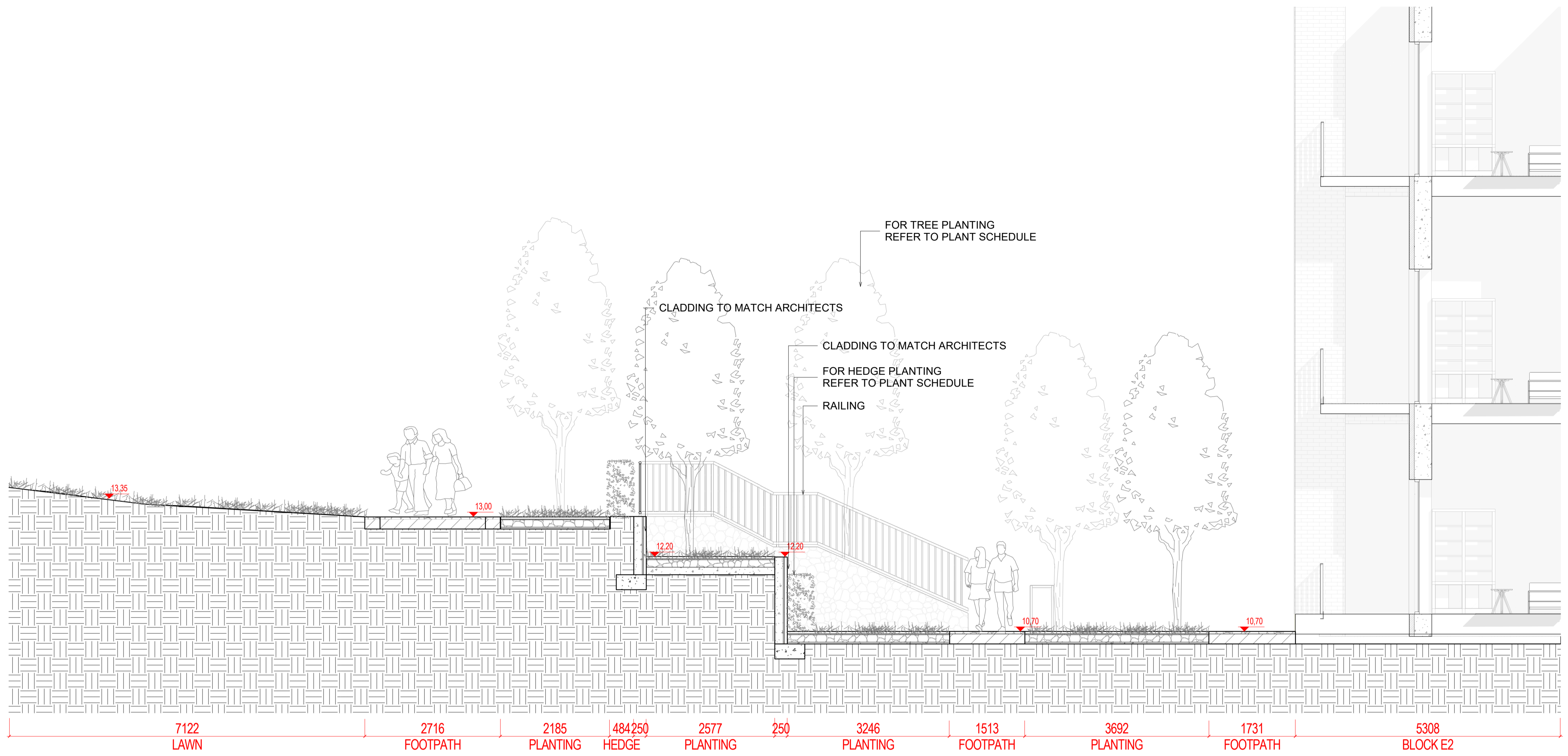
1 SECTION 70 1:50 @A1
