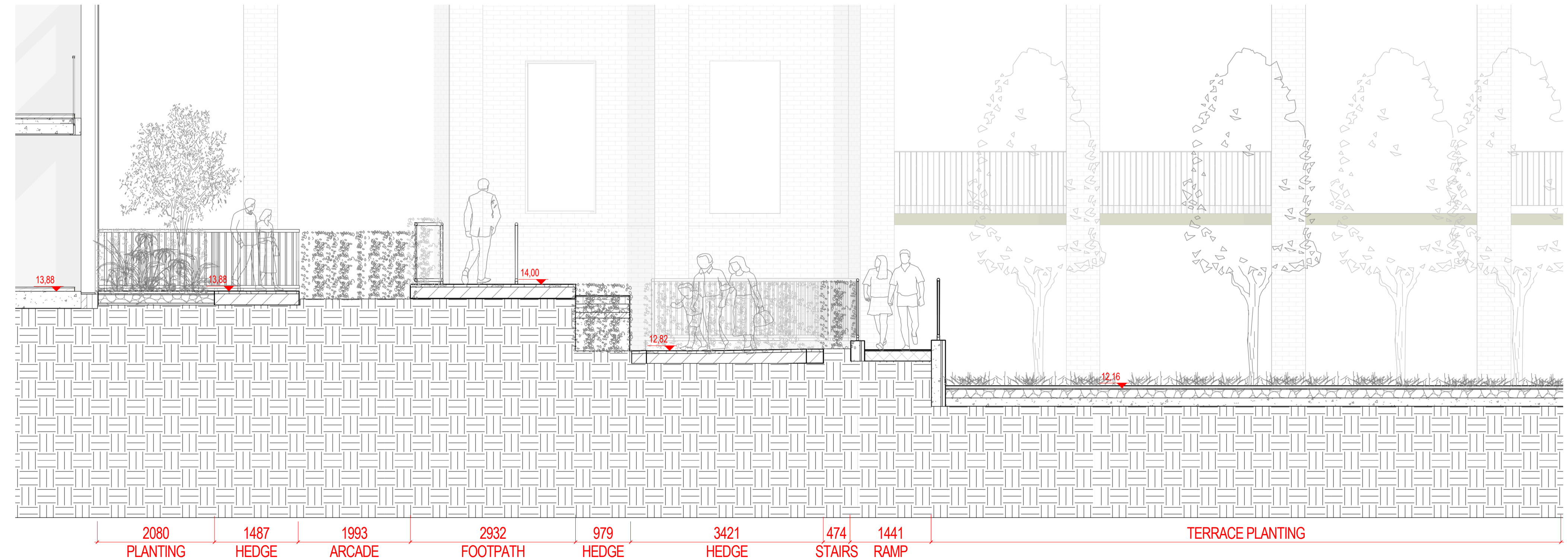
2 SECTION 71 1:50 @A1
